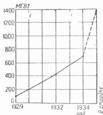
Рис. 44. Рост суммарной мощности гидроэлектростанций СССР.
