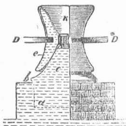
Рис. 19. Римская ручная мельница.
