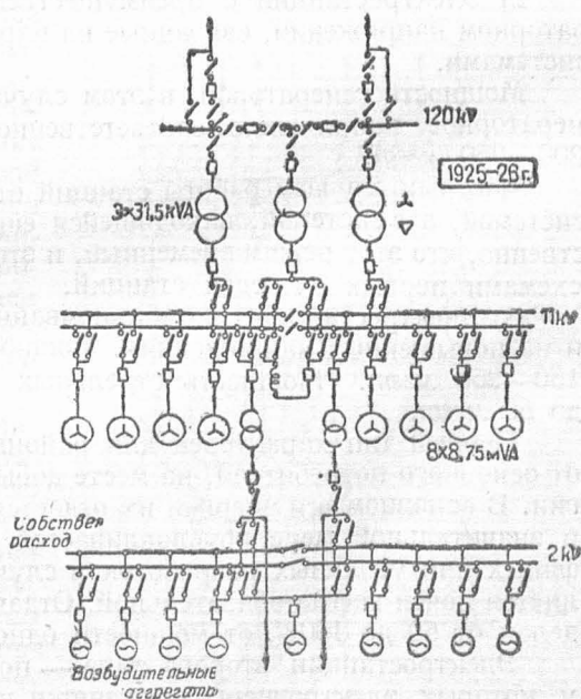
Рис. 10. Схема Волховской ГРЭС 1925—1926 гг.
