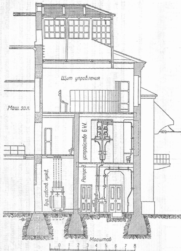
Рис. 27. Распределительные устройства 6 кВ Горьковской ГРЭС. Слева — старое, справа — новое.
