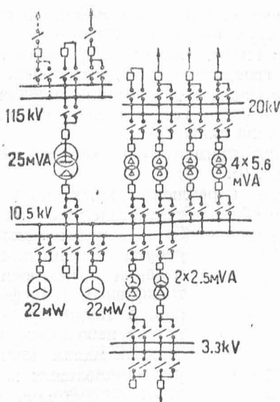
Рис. 5. Схема первой очереди ГРЭС им. Артема 1928—1929 гг.
