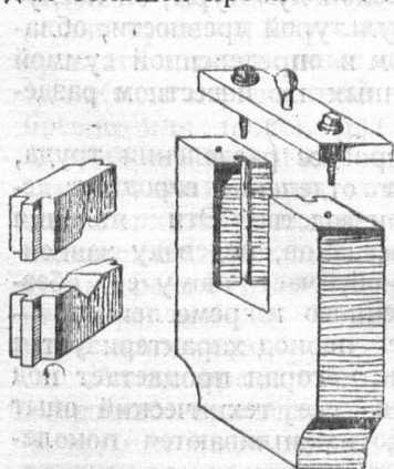
Рис. 4. Разъемный подшипник токарного станка со вставными деревянными вкладышами, допускающий подтяжку по мере износа. Начало XVIII в.
