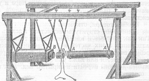
Рис. 5. Аппарат для определения механического эквивалента по способу Гирна.
