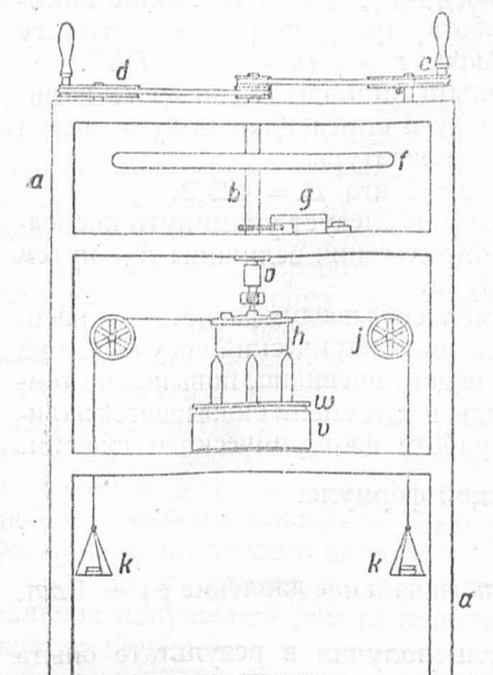
Рис. 3. Усовершенствованный аппарат Джоуля.
