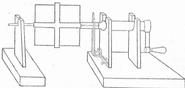
Машина Фарадея с прямоугольным контуром, вращающимся в магнитном поле земли.
