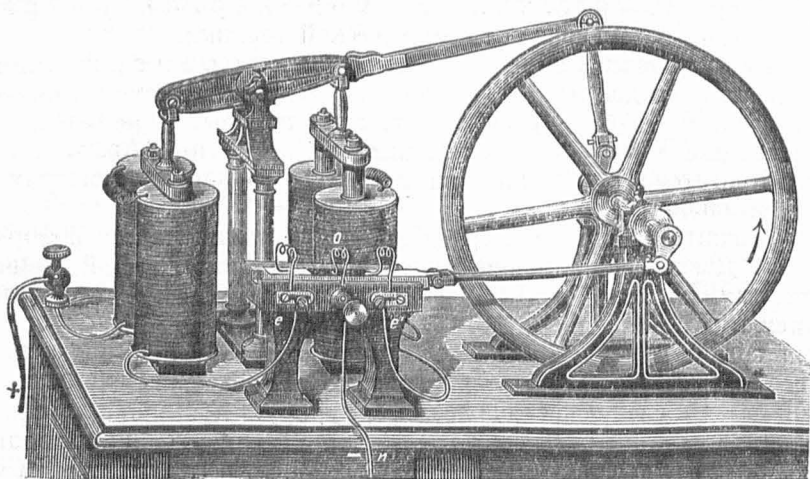
Двигатель Бурбуза.
