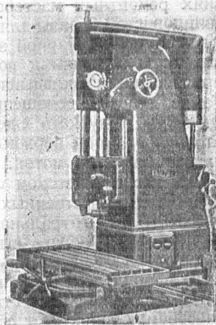
Рис. 20. Вертикальный станок для чистовой расточки (Feinbohren) фирмы «Краузе». Скорость: до 3 000 об/мин, подача до 0,01 мм.
