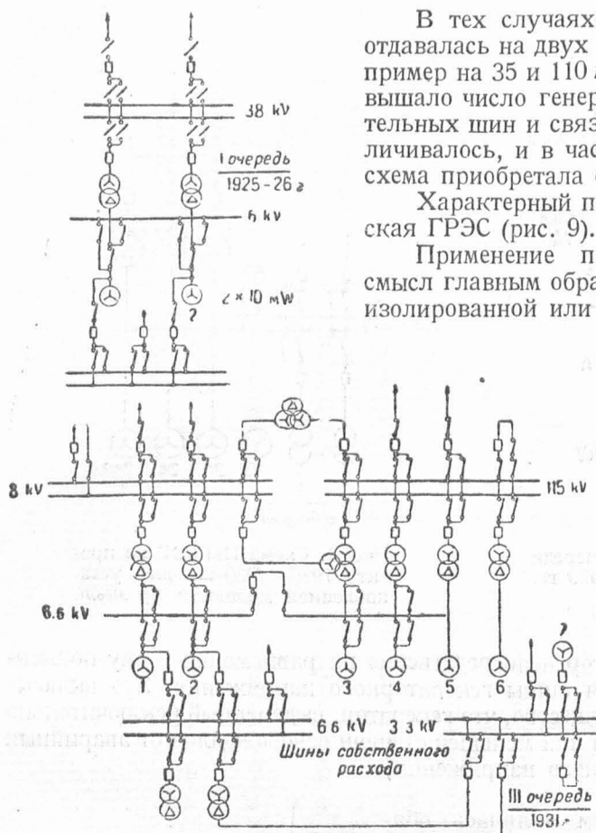
Рис. 8. Развитие схемы Штеровской ГРЭС.
