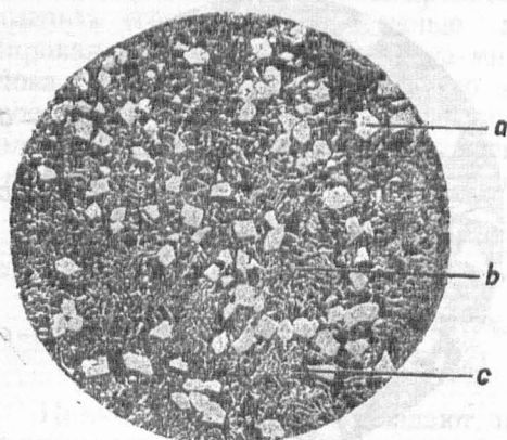
Рис. 11. Микроструктура свинцового баббита, содержащего 5% олова; 15% Sb и остальное свинец.
