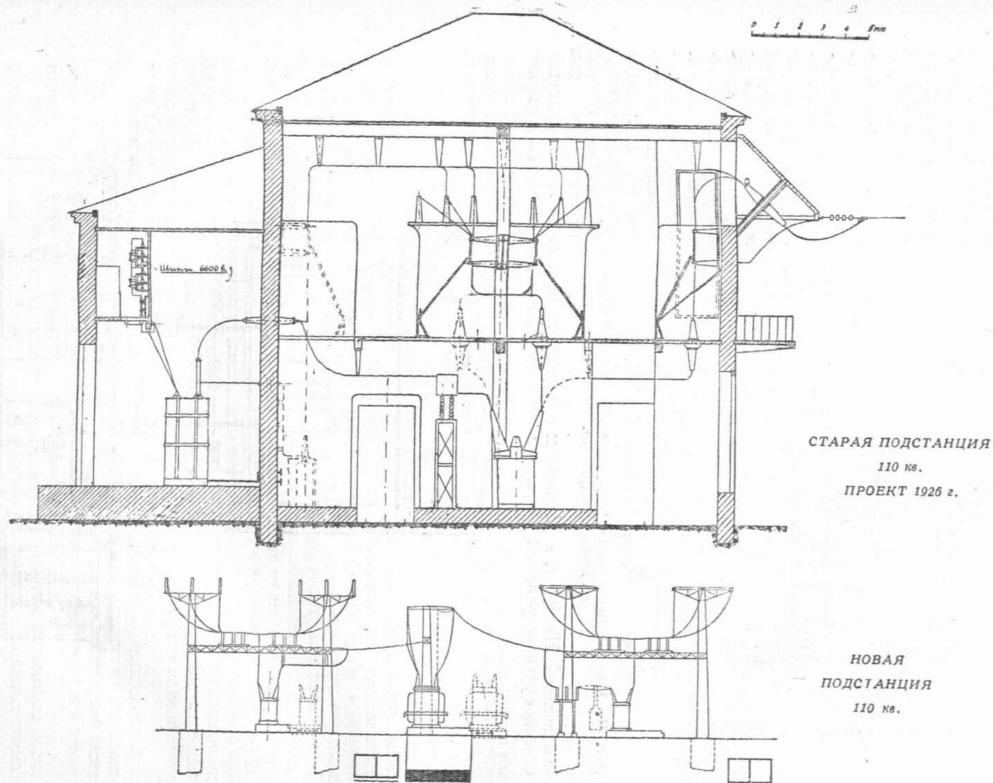
Рис. 30. Повысительные подстанции 110 кв Горьковской ГРЭС.
