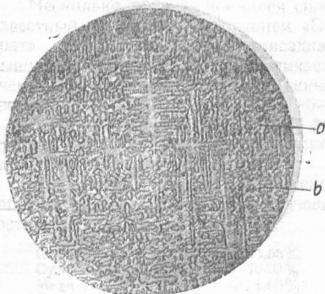
Рис. 9. Микроструктура литой оловянистой подшипниковой бронзы, содержащей 10% олова.
