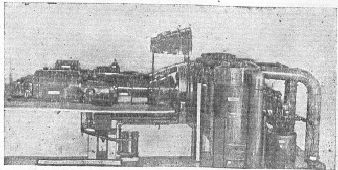
Рис. 6. Паровой турбогенератор в 50 000 кет (построен в 1924 г. на заводах Парсонса).
