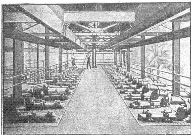
Рис. 8. Платформа батареи № 4 на заводе в Аскерне, с которой производится загрузка угля в реторты. Видны верхушки реторт и газоходы.
