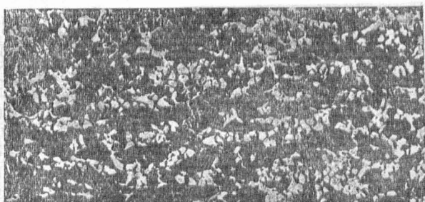
Рис. 19. Микроструктура свинцовой бронзы, содержащей 45% Pb, 0,4% серы и 1,5% кремнецирконового сплава.
