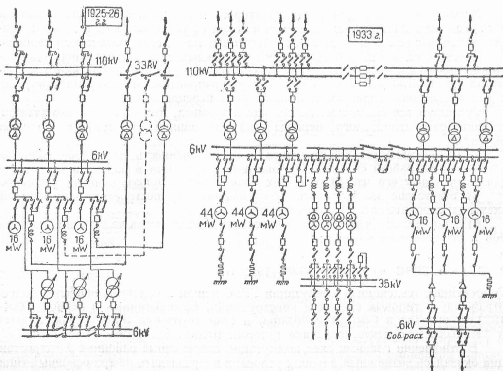
Рис. 9. Развитие схемы Шатурской ГРЭС им. В. И. Ленина.
