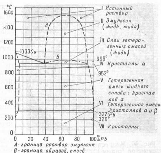
Рис. 15. Диаграмма состояния медно-свинцовых сплавов по В. Клаусу (W. Claus).
