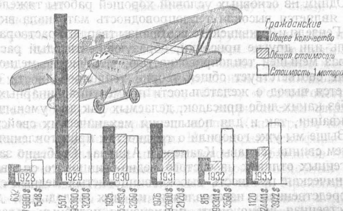
Рис. 14а. Статистика производства гражданских авиамоторов в США (по Aircraft Year book for 1934).
