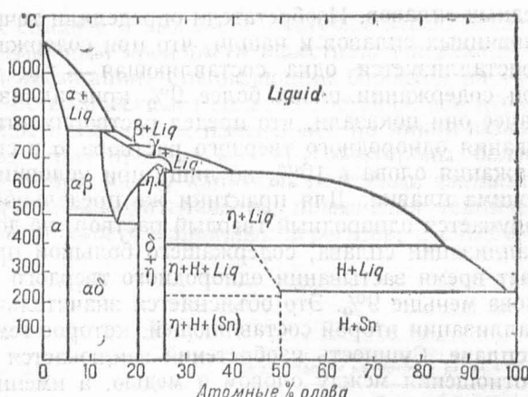
Рис. 6. Диаграмма состояния медно-оловянных сплавов, опубликованная в 1903 г. исследователями Heuscock и Neville.
