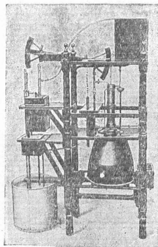
Рис. 3. Модель «атмосферной машины».
