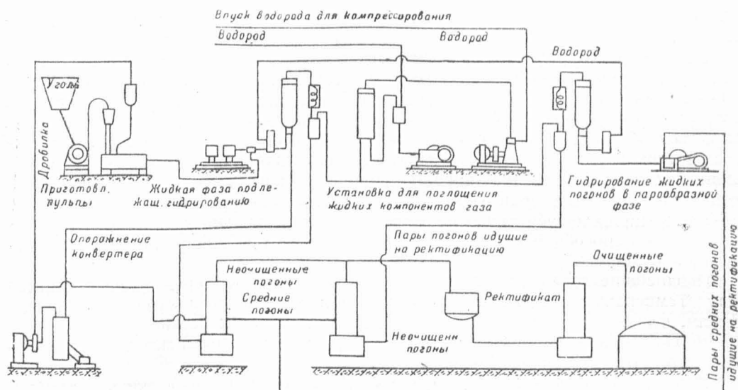
Рис. 9. Схема расположения аппаратуры и циркуляции продуктов на установке для гидрирования угля в Билинге (Англия).
