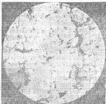
Рис. 16. Микроструктура литой свинцовой бронзы (30% Pb), полученная при медленном охлаждении. Свинец ликвирован и распределен неравномерно. Шлиф не травлен.
