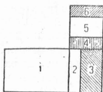
А. Каширская ГРЭС 1921—1922 гг.
