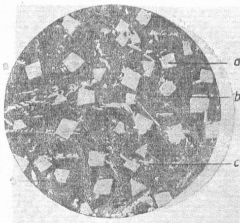
Рис. 10. Микроструктура нормального баббита, содержащего: 5—6% меди; 12—13% сурьмы; остальное олово.
