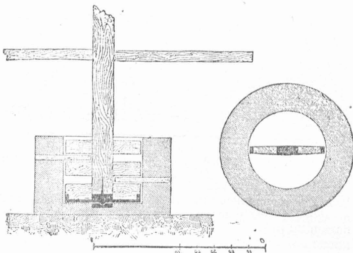
Рис. 21. Римская тестомесилка в I в. н. э.
