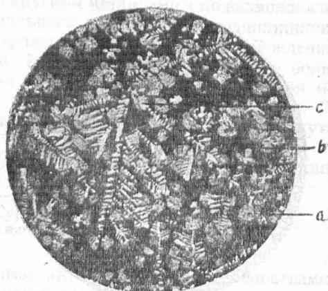
Рис. 12. Микроструктура лурги-металла.
