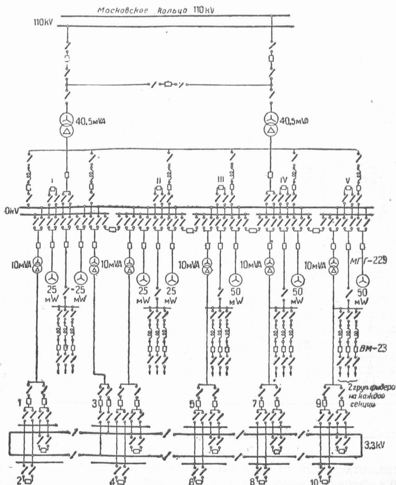
Рис. 15. Схема полного развития Сталинской ТЭЦ (Москва).
