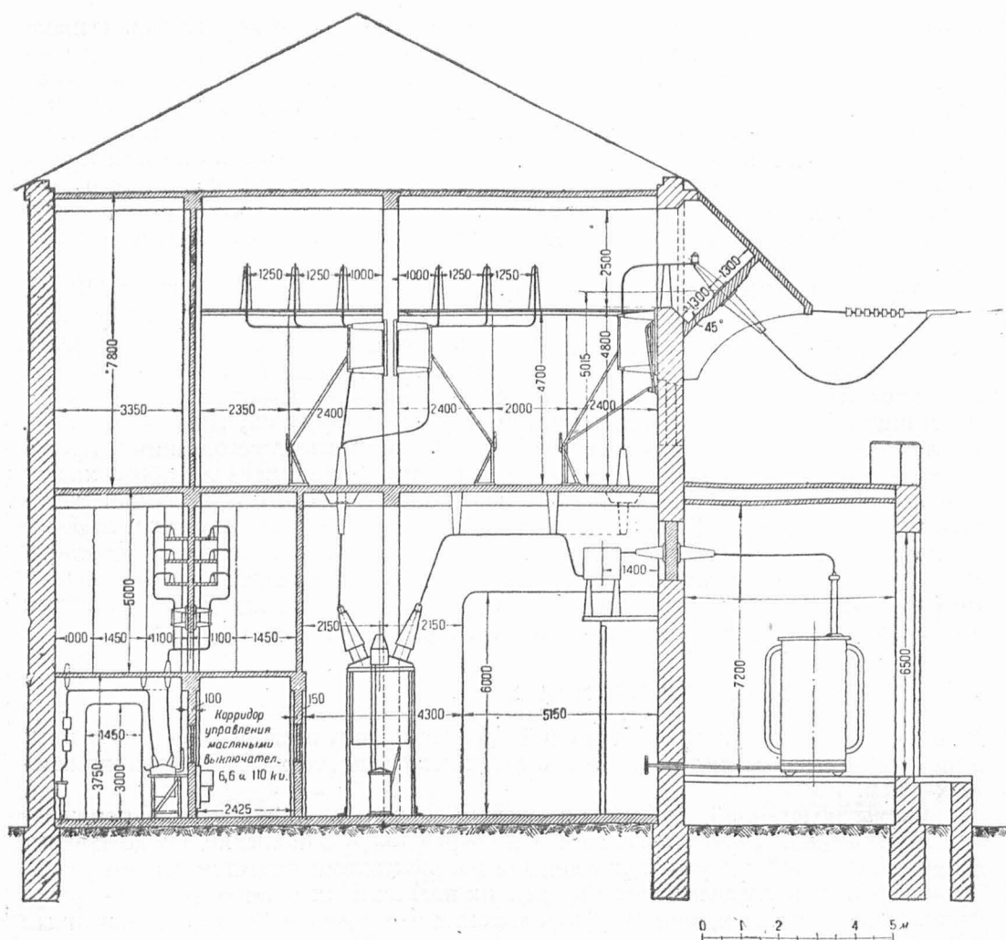
Рис. 36. Понижительные подстанции в Сормове и Молитовке, 110/6 кВ (сеть Горьковской ГРЭС).
