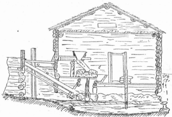
Рис. 20. Греческая водяная мельница в I в. н. э.
