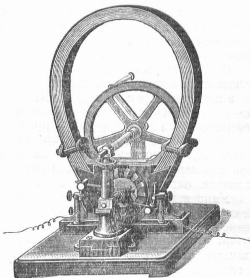
Машина Грамма.
