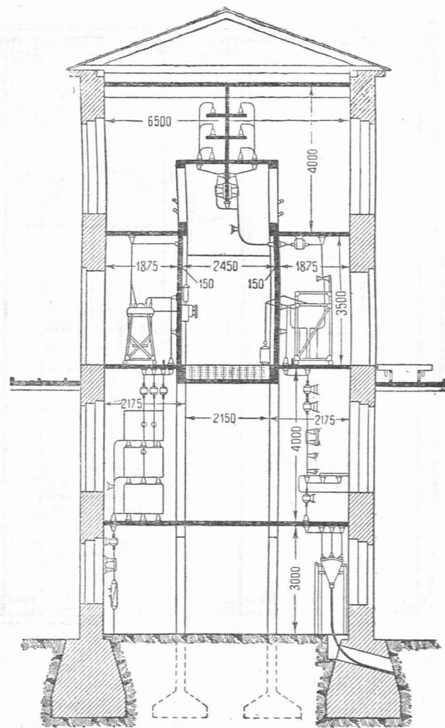
Рис. 27. Распределительные устройства 6 кВ Горьковской ГРЭС. Слева — старое, справа — новое.
