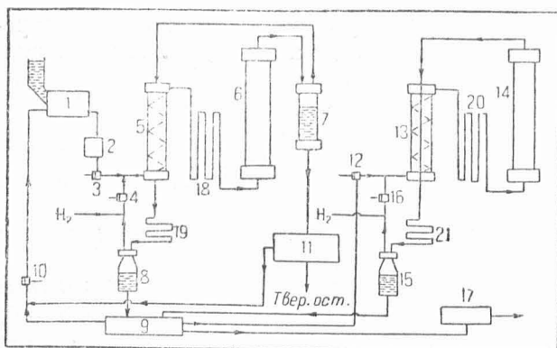
Рис. 2. Схема процесса гидрирования угля на заводе «И. Г. Фарбениндустри» в Леуна.
