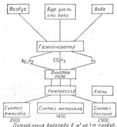
Рис. 10. Схема синтеза аммиака, метанола и бензина на заводе «И. Г.» в Леуна.
