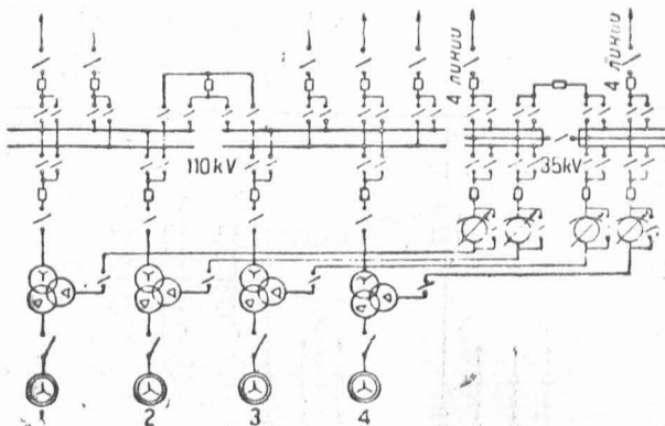
Рис. 13. Схема Дубровской ГРЭС (Ленэнерго).
