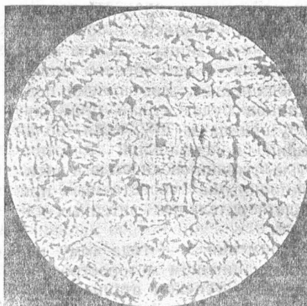
Рис. 17. Микроструктура литой свинцовой бронзы (30% Pb), полученная при интенсивном охлаждении. Свинец распределен равномерно, не нарушая непрерывности сетки медных кристаллов. Шлиф не травлен. Увеличение \times 100 .
