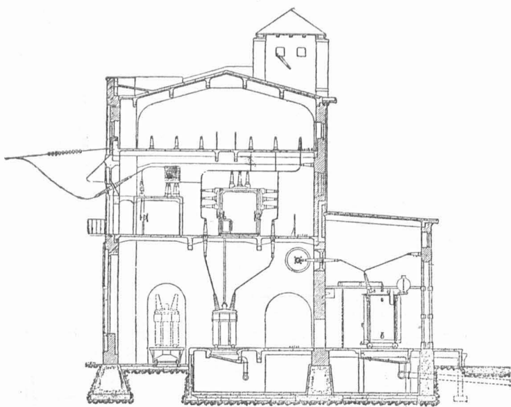
Рис. 31. Понижительная подстанция 110 кВ Волховской ГРЭС в Ленинграде (разрез).
