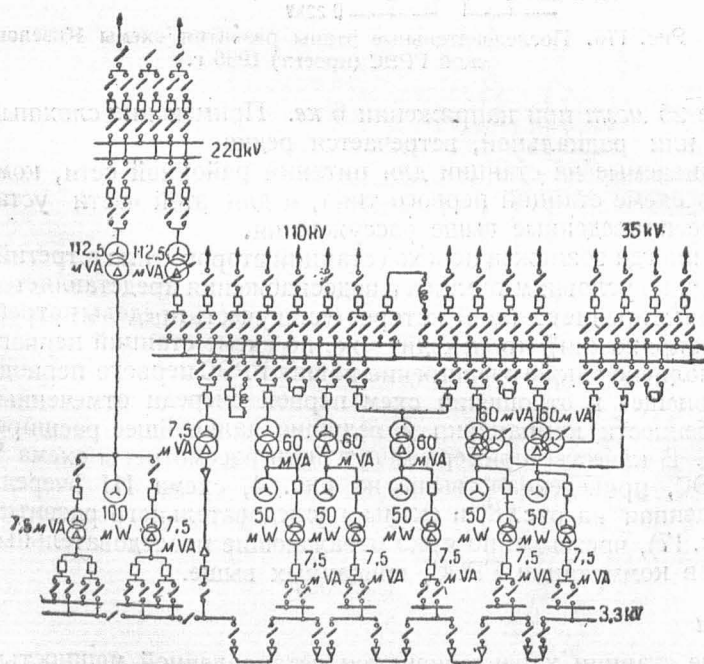
Рис. 19. Один из вариантов расширения Зуевской ГРЭС до 350 мвт (Теплоэлектропроект).
