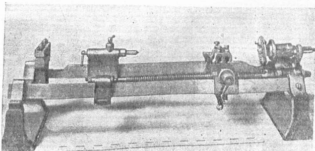
Рис. 15. Токарно-винторезный станок Модслея (1800 г.).
