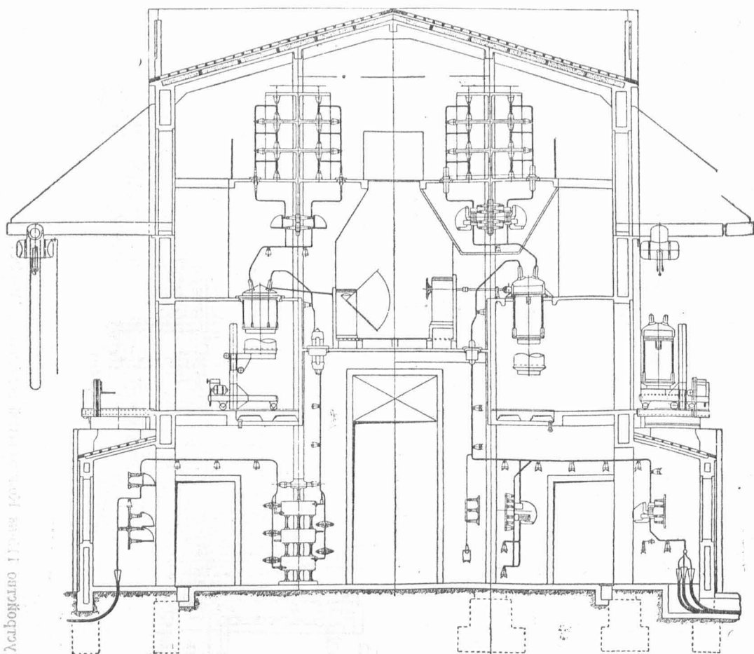
Рис. 38. Распределительное устройство 6-кв Сокольнической подстанции Московского кольца 110 кв.
