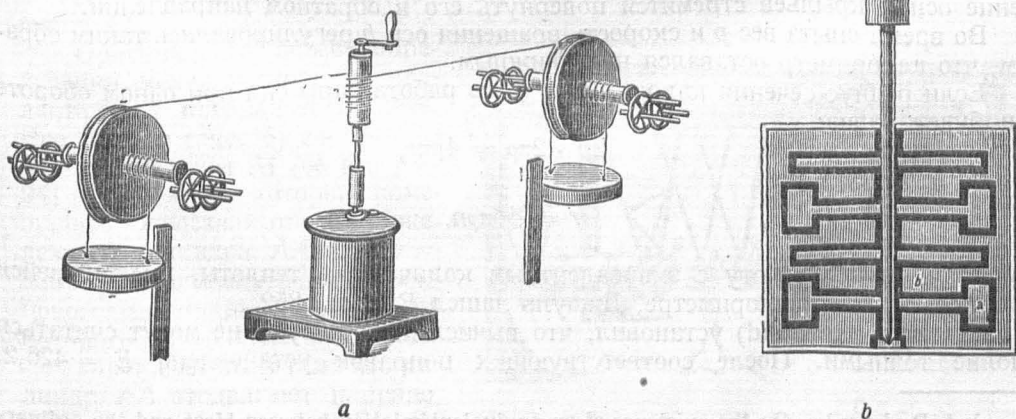
Рис. 1. а — прибор для опыта Джоуля; б — лопатки прибора для опыта Джоуля.
