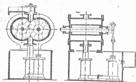
Рис. 5. Проект ротативного парового двигателя Мурдоха 1799 г., представляющего по своей конструкции копию водоподъемного ротативного насоса „Machina Parrenhemiana“ XVII в.
