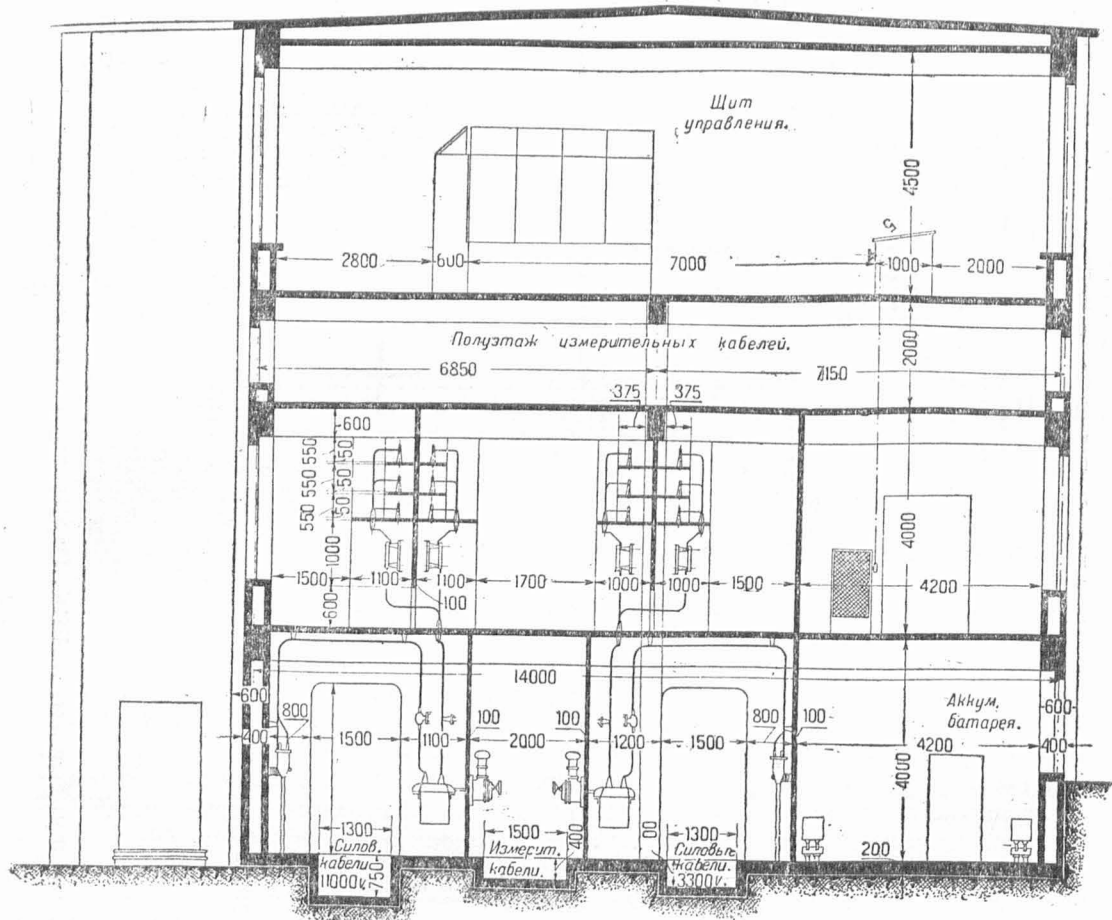
Рис. 28. Распределительное устройство
