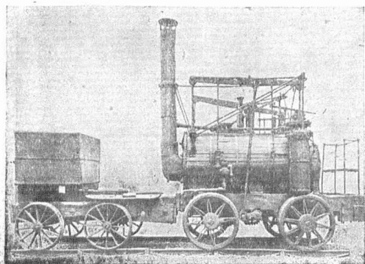
Рис. 7. Старейший локомотив «Пыхтящий Билли» (построен Хидлеем в 1813 г.).
