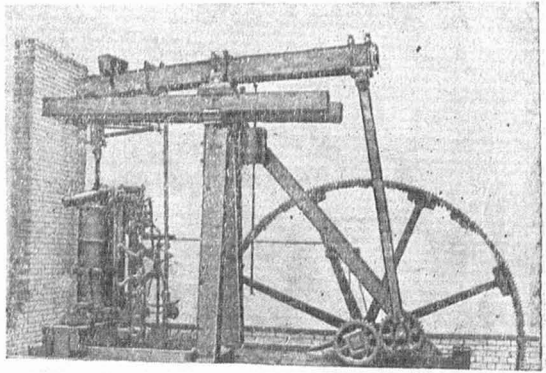
Рис. 4. Паровая машина Джемса Уатта (с планетарным механизмом). Построена в 1788 г.
