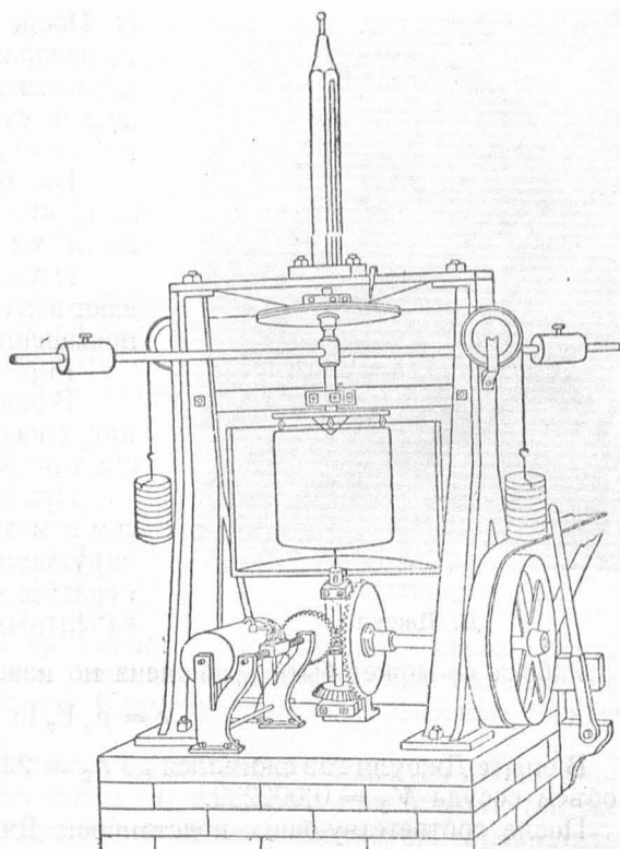
Рис. 4. Прибор для определения механического эквивалента, работающий от нефтяного двигателя.
