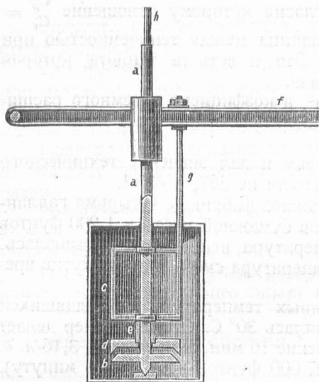
Рис. 2. Прибор для определения механического эквивалента путем трения чугуна.
