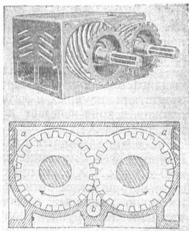
Рис. 8. Турбина Спиро, приводимая в движение сжатым воздухом.
