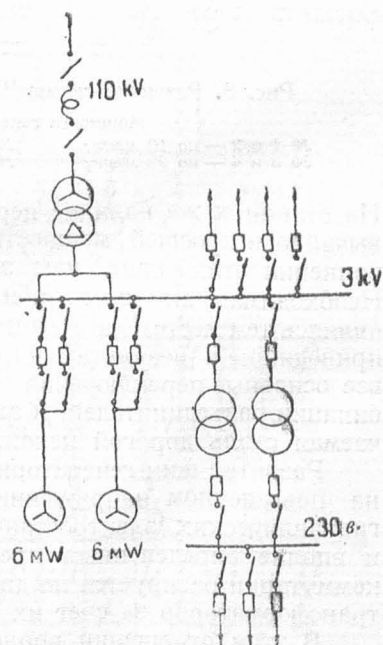
Рис. 7. Схема Каширской ГРЭС 1921—1922 гг.
