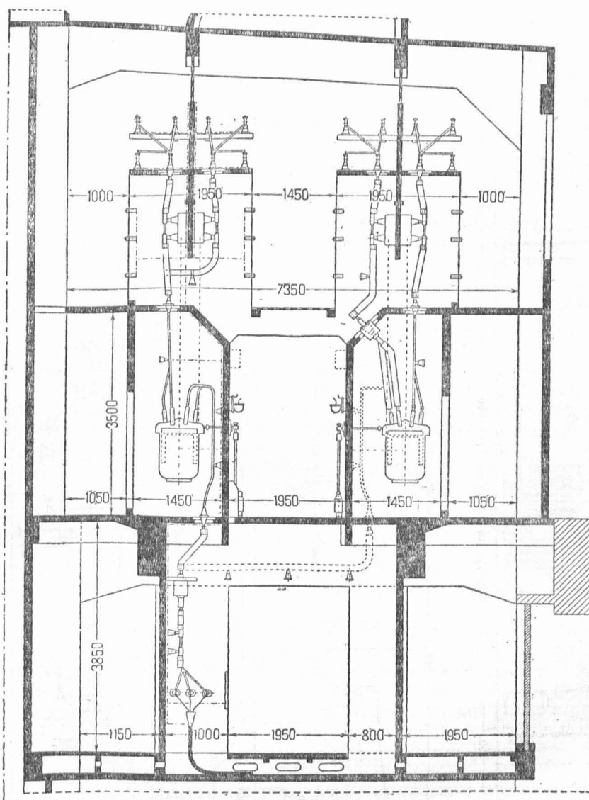
Рис. 34. Камеры трансформатора 10 мвга и соединительного масляного выключателя распределительного устройства 3 кв Сталинской ТЭЦ.
