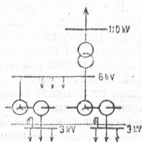
Рис. 22. Принципиальная схема питания собственного расхода станции вспомогательными генераторами, сидящими на валу главных турбин.
