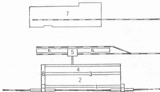
Рис. 26. Более позднее решение ситуационной компоновки ГРЭС (проект Магнитогорской ЦЭС).
