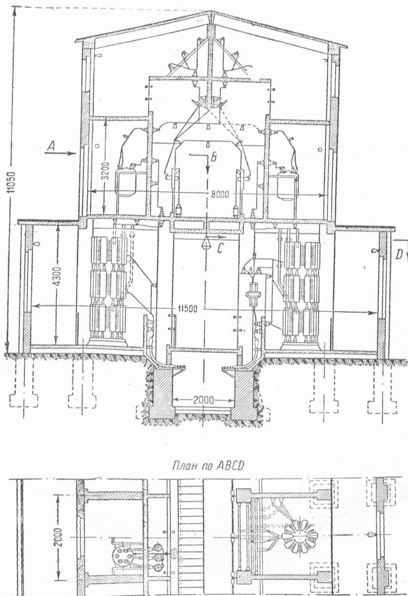
Рис. 39. Разрез распределительного устройства подстанции 6 кВ реакторного типа по стандарту 1933 г. (Теплоэлектропроект).
