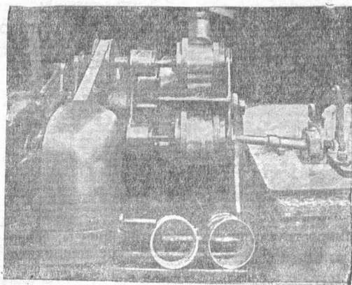
Рис. 21. Высокопроизводительный четырехшпиндельный центробежный станок для заливки подшипников баббитом. Производительность 100 подшипников в час. Толщина слоя заливки от 1,5 до 2,5 мм.
