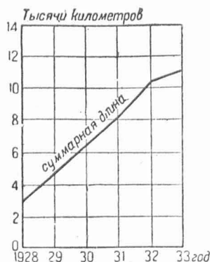
Рис. 42. Рост протяженности высоковольтных сетей СССР.
