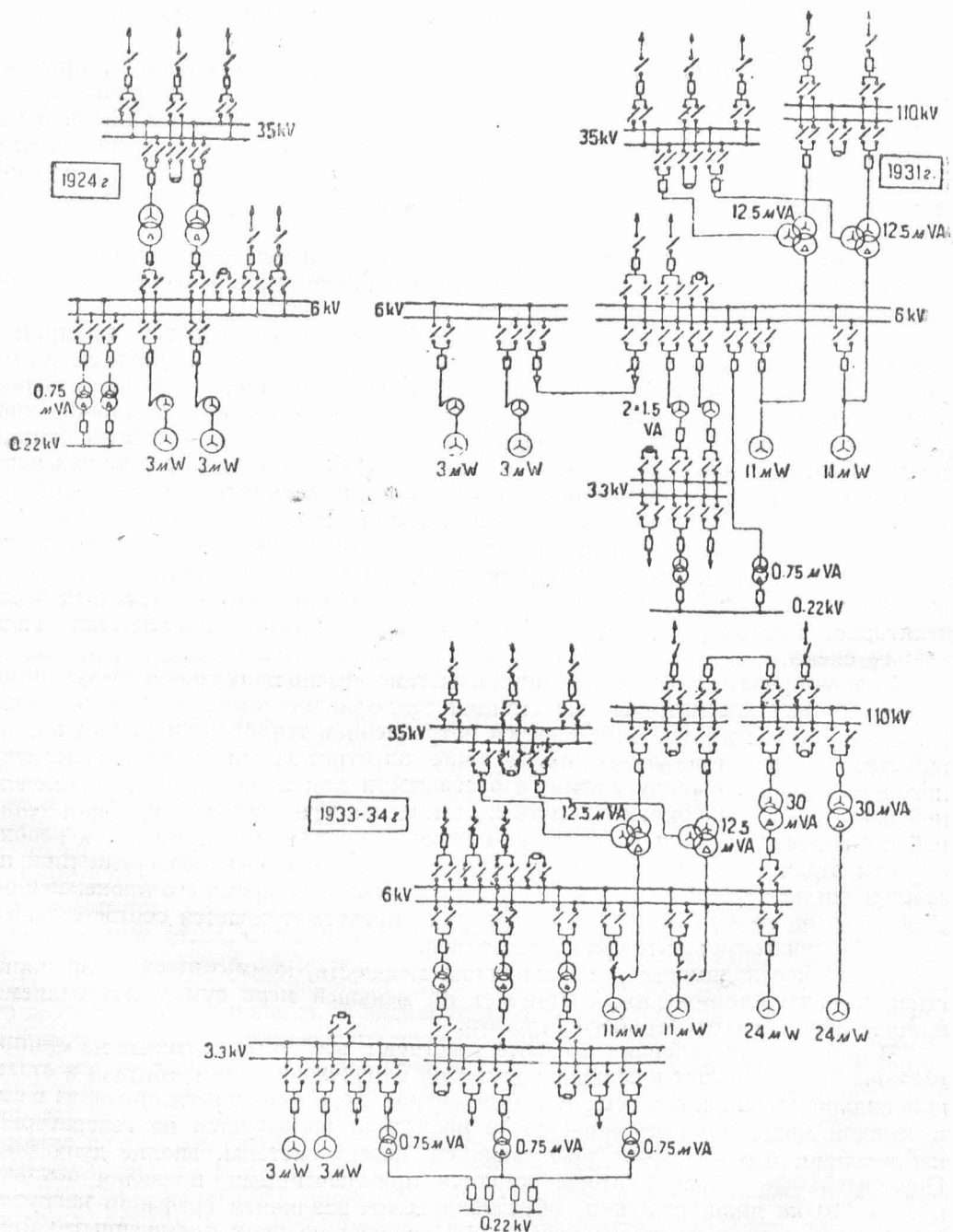
Рис. 17а. Последовательные этапы развития схемы Кизеловской ГРЭС (проект) 1924, 1931, 1933—1934 гг.
