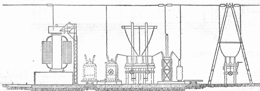
Рис. 29. Распределительные устройства 35 кв Горьковской ГРЭС.
