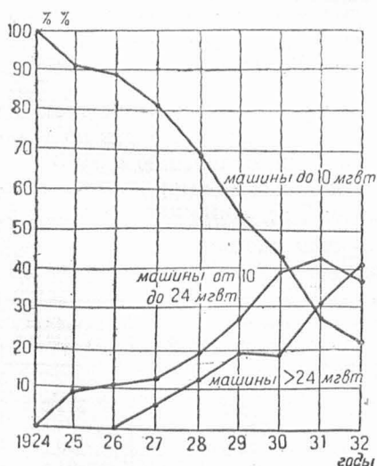
Рис. 43. Динамика удельного веса генераторов различной мощности на районных станциях СССР.
