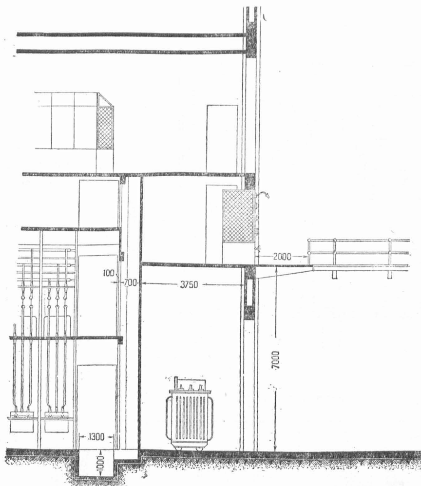
ство 10 кВ ГРЭС им. Артема.
