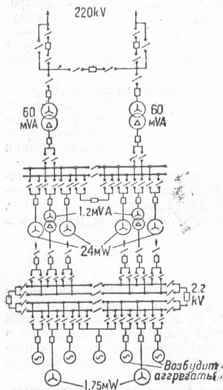
Рис. 12. Свирская ГРЭС (схема полного развития).
