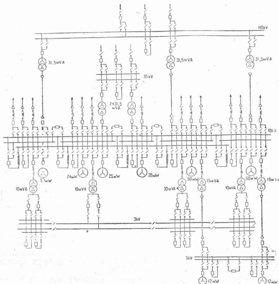
Рис. 14. Магнитогорская ЦЭС (проект схемы полного развития, ТЭЦ).
