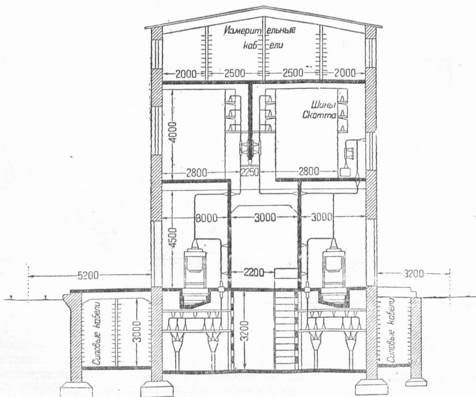
Рис. 32. Распределительное устройство 10 кВ Магнитогорской ЦЭС.
