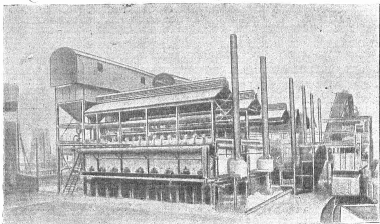
Рис. 7. Вид шести батарей реторт для полукоксования углей на заводе в Аскерне (Англия). Слева над батареей реторт видна приемная эстакада, с которой производится загрузка бункеров. Справа видна установка для отсеивания полукоксовки и его погрузки.
