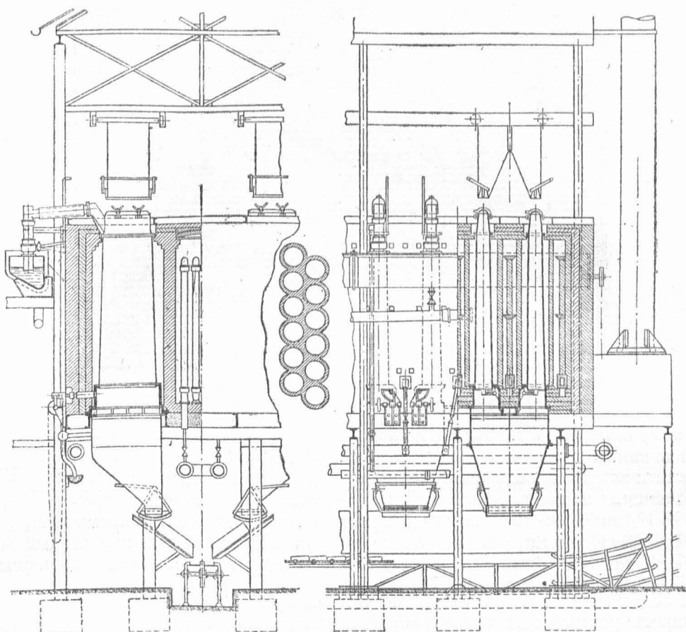
Рис. 6. Схема реторт для полукоксования углей на заводе в Аскерне (Англия). Слева показана реторта, над которой находится бункер, служащий для загрузки ее углем. В центре дается, в разрезе сверху, трубчатая конструкция реторты. Справа видны две реторты, внизу которых помещены камеры для охлаждения полукокса, а сверху — бункера для загрузки.
