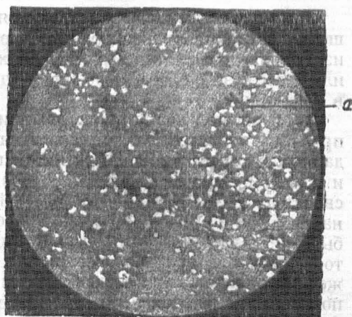
Рис. 13. Микроструктура гиттер-металла состава: 5% меди; 7—8% сурьмы; 0,14% углерода; остальное олово.
