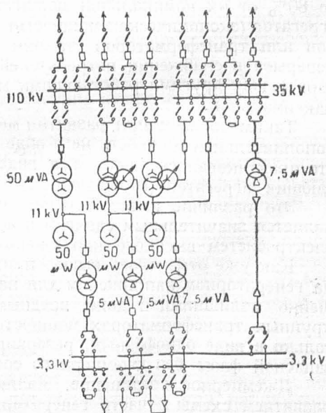
Рис. 11. Схема Зуевской ГРЭС 1931 г.
