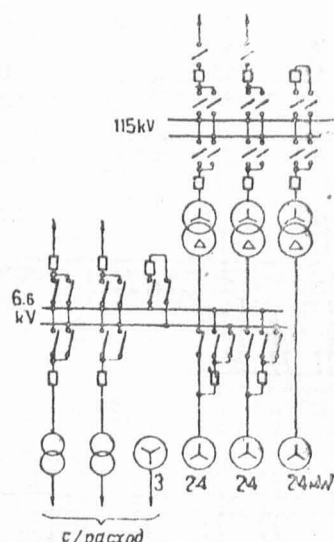
Рис. 6. Схема ИвГРЭС по проекту 1929—1930 гг. для установленной мощности 75 мвт.
