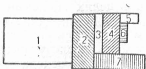
Б. ГРЭС «Красный Октябрь» 1923—1924 гг.
