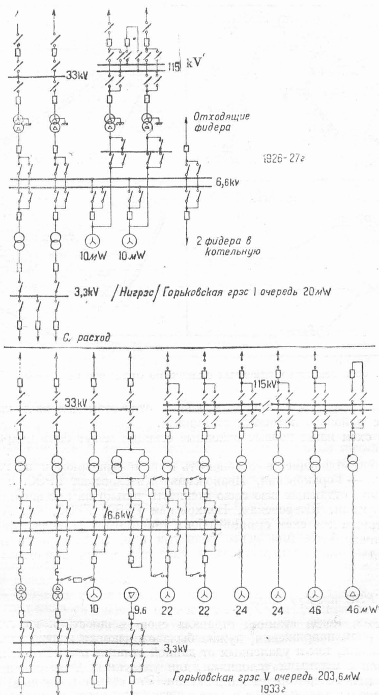
Рис. 4. Схемы отдельных этапов развития Горьковской ГРЭС.
