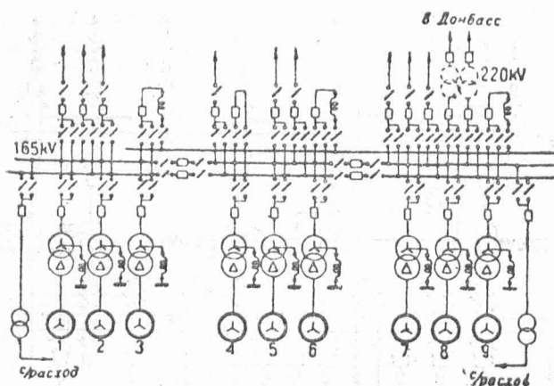
Рис. 18. Схема Днепровской ГРЭС им. В. И. Ленина. Генераторы 1—9 по 62 мвт. Повысительные трансформаторы 9 \times 78 мва; 13,2/160 кв. Трансформаторы собственного расхода 2 \times 6 мва; 160/2,7 кв.
