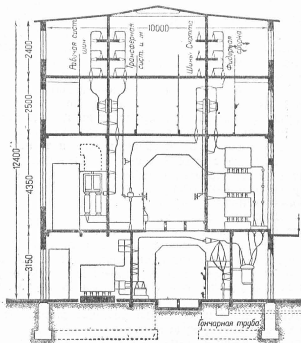
Рис. 33. Камеры группового и отходящего фидеров распределительного устройства 10 кв Сталинской ТЭЦ (Москва).
