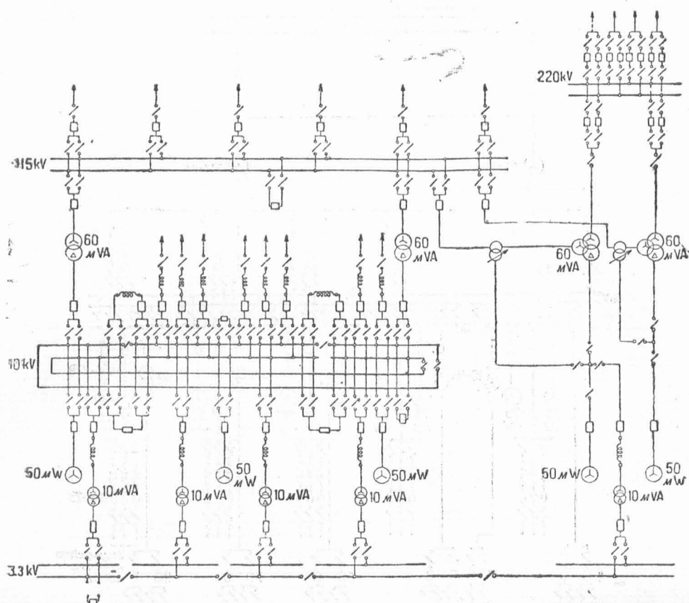
Рис. 16. Сталиногорская (Бобриковская) ГРЭС им. Сталина для мощности 250 мвт.
