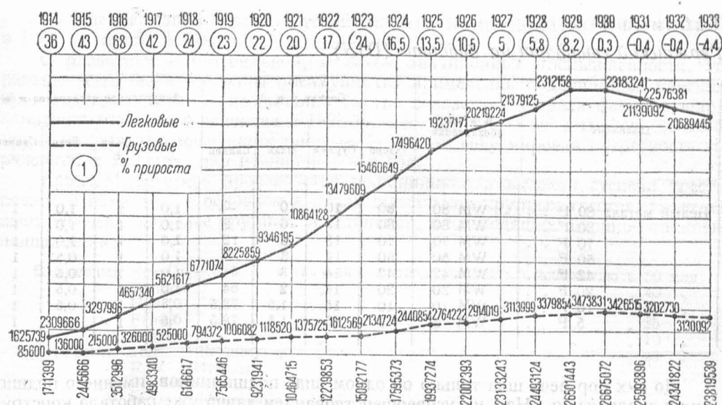
Рис. 8. Кривая регистрации новых автомобилей в США (по данным департамента коммерции США и журнала «Automotive Industries»).
