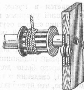
Рис. 3. Деревянный подшипник, обитый железом. XVI в.
