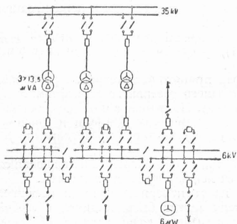
Рис. 23. Схема питания собственного расхода Дубровской ГРЭС.
