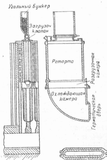
Рис. 1. Реторта для полукоксования углей на опытной установке фирмы «Лоу Темперачюр Карбонизейшен».
