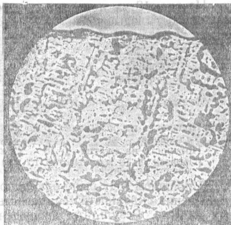
Рис. 18. Микроструктура вкладыша, залитого свинцовистой бронзой, американской фирмы «Allison» (30% Pb). Место спая бронзы со сталью. Кристаллы меди «растут» от стали к рабочей поверхности. Шлиф не травлен.
