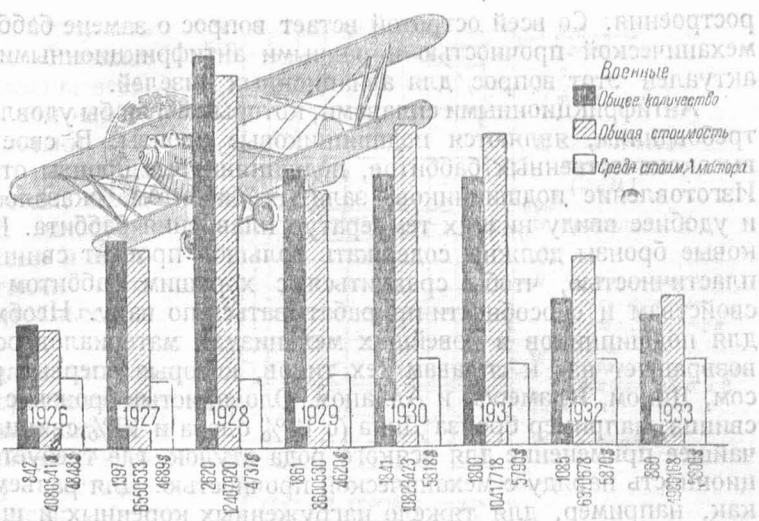
Рис. 14. Статистика производства военных авиамоторов в США (по Aircraft Year book for 1934).
