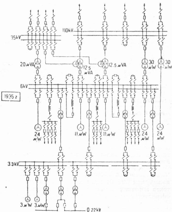
Рис. 176. Последовательные этапы развития схемы Кизеловской ГРЭС (проект) 1935 г.
