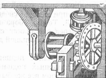
Рис. 2. Висячий подшипник, окованный железной скобой для прочности. Относится к XVI в.
